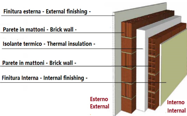
Esempio della struttura di una parete (stratigraphy) Example of the structure of a wall (stratigraphy)
