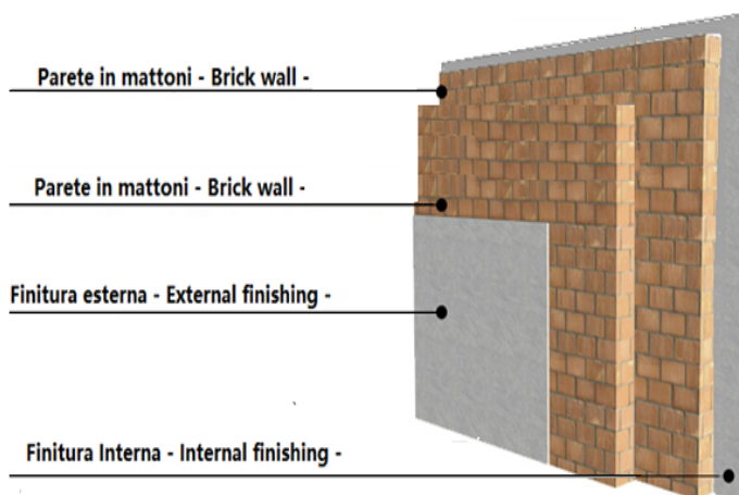
Esempio della struttura di una parete (stratigraphy) Example of the structure of a wall (stratigraphy)
